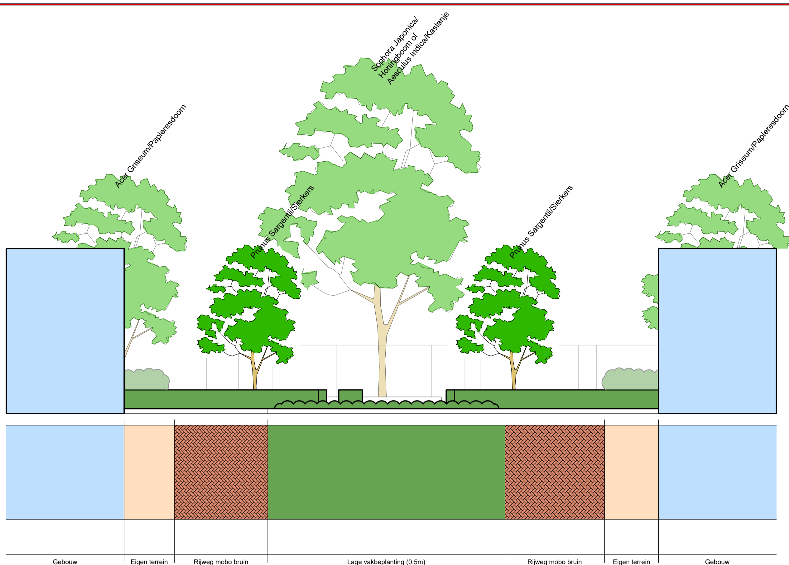
A-A' Aanzicht vanaf entree Fazantenveld
